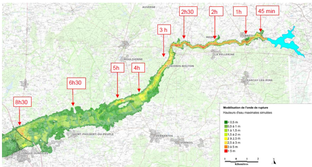
Figure 3: Risque de rupture du barrage des Mousseaux (source: SAFEGE)
