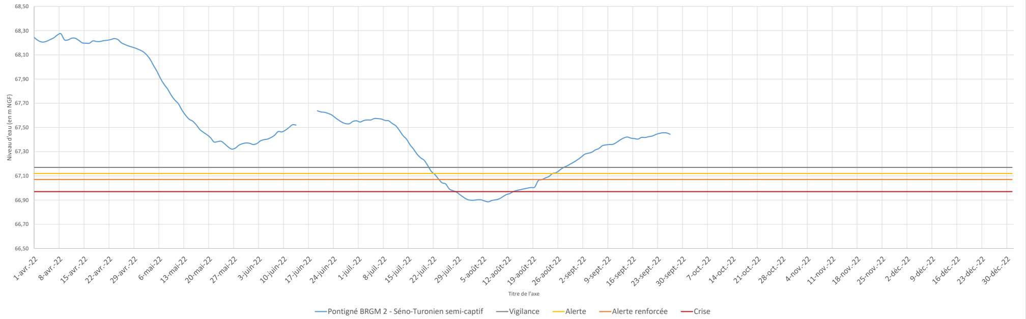
Évolution du niveau de la nappe à Pontigné BRGM 2 - Séno-Turonien semi-captif (04248X0022/F) et seuils d'alerte
